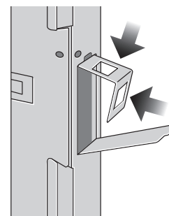
2.) Darunterliegende, zweifach gelochte Stabhalterung, kreisbogenförmig herausziehen und mittig knicken, sodass die Löcher deckungsgleich übereinander liegen.
