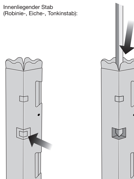
3.) Verschlusslaschen mit schneller Bewegung und Druck in die Ausstanzungen der Verriegelung drücken.
