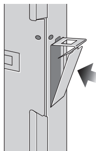
3.) Verschlusslasche wieder nach oben in die Wandung drücken um das rechteckige Loch unter der entstandenen Stabhalterung zu schließen. Mit der zweiten Stabhalterung, wie vorstehend beschrieben, verfahren.
